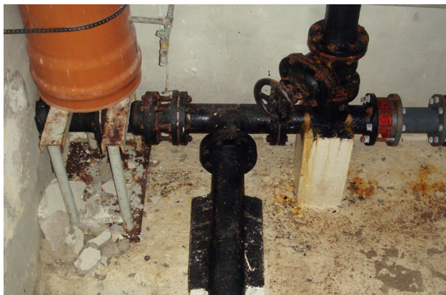
Fig. 3 : Moisture penetration damage
